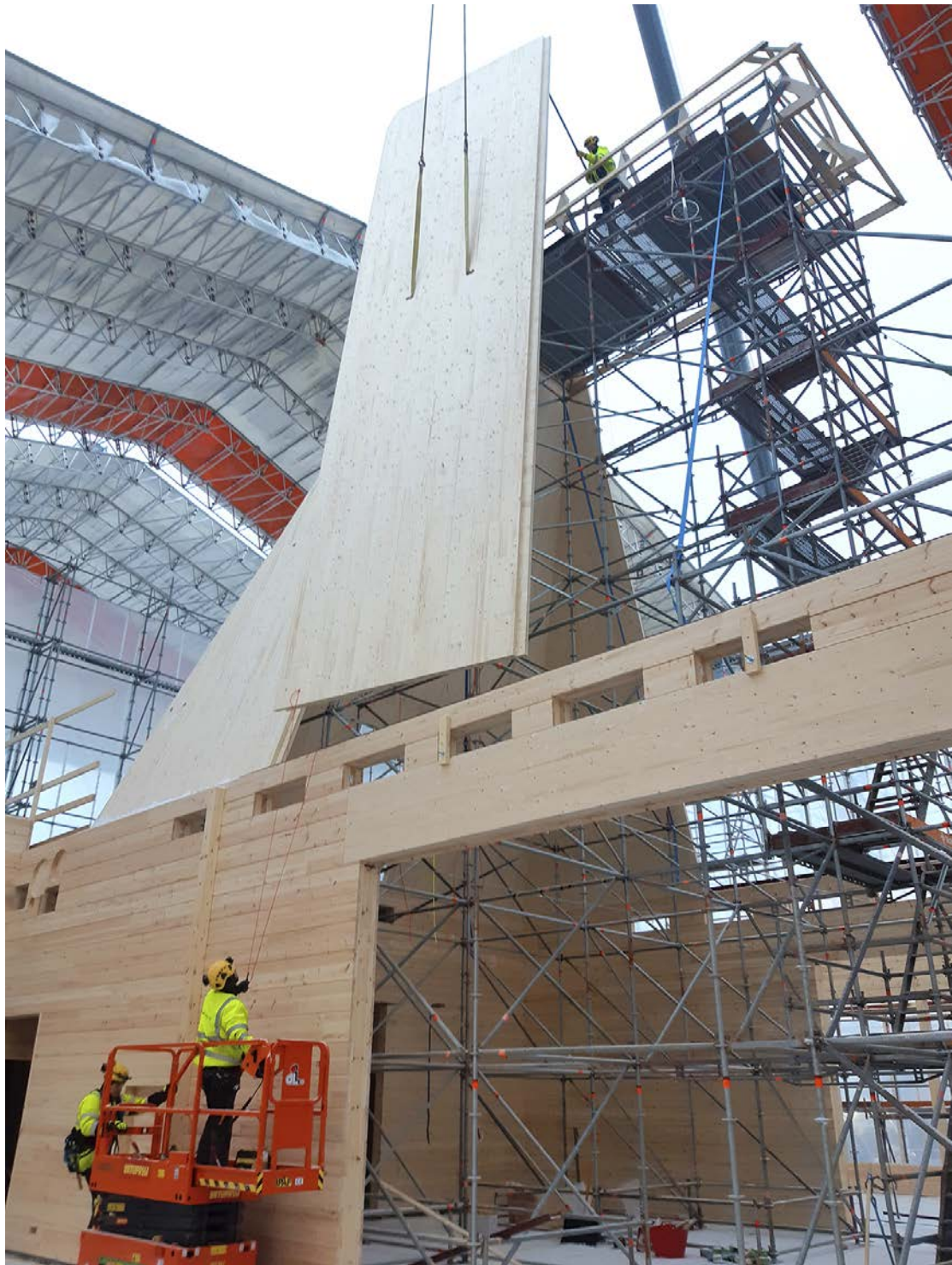
Kirkon hirsirunko on jo valmis. Joulukuun puolivälissä rakennuksella alettiin asentaa kirkon yläpohjan CLT-monikerroslevyjä.
